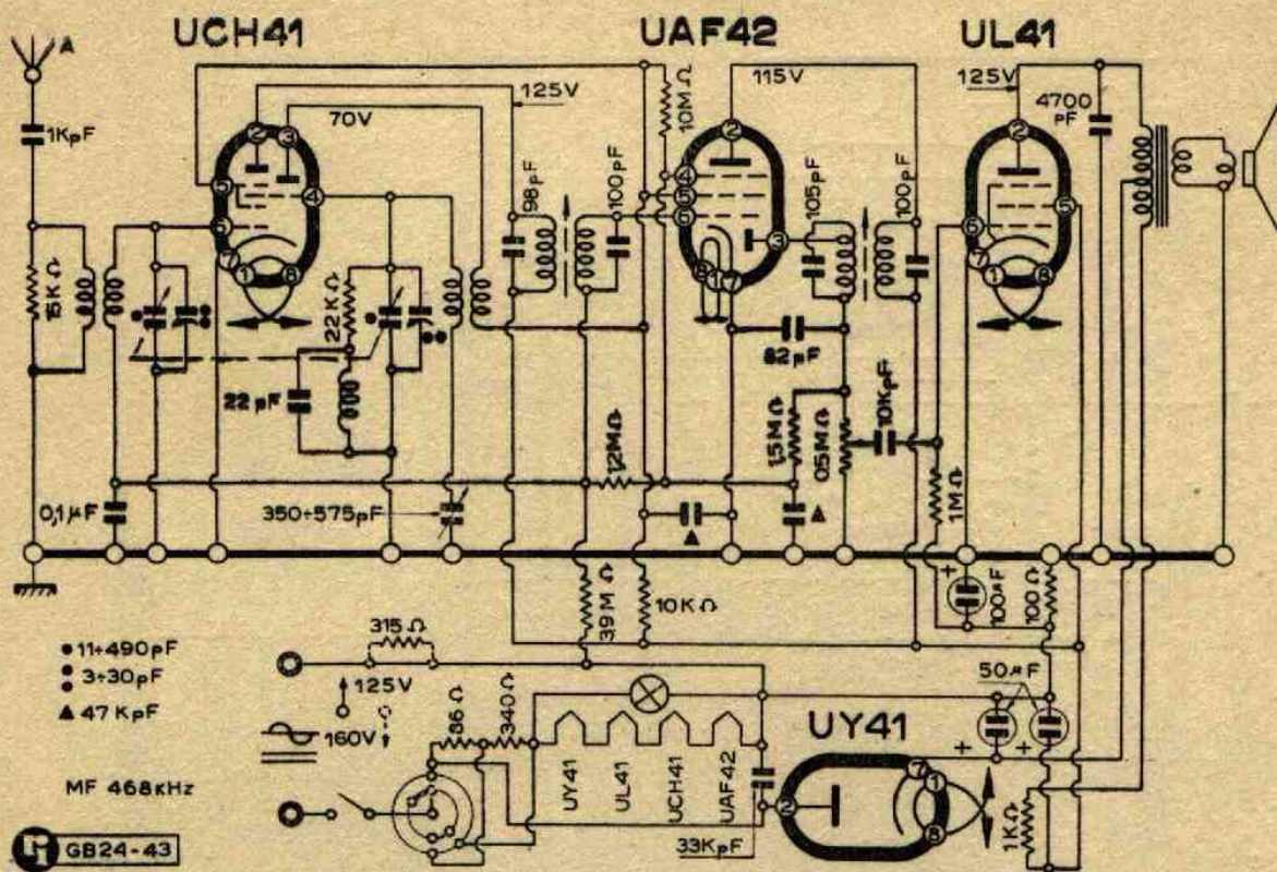
Lo schema elettrico del mod. BI 190 U
